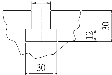
T型溝尺寸詳圖
