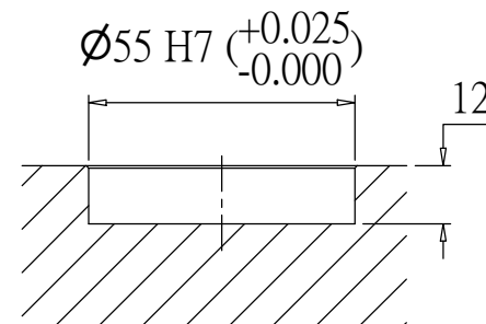
盤面中心孔剖面
